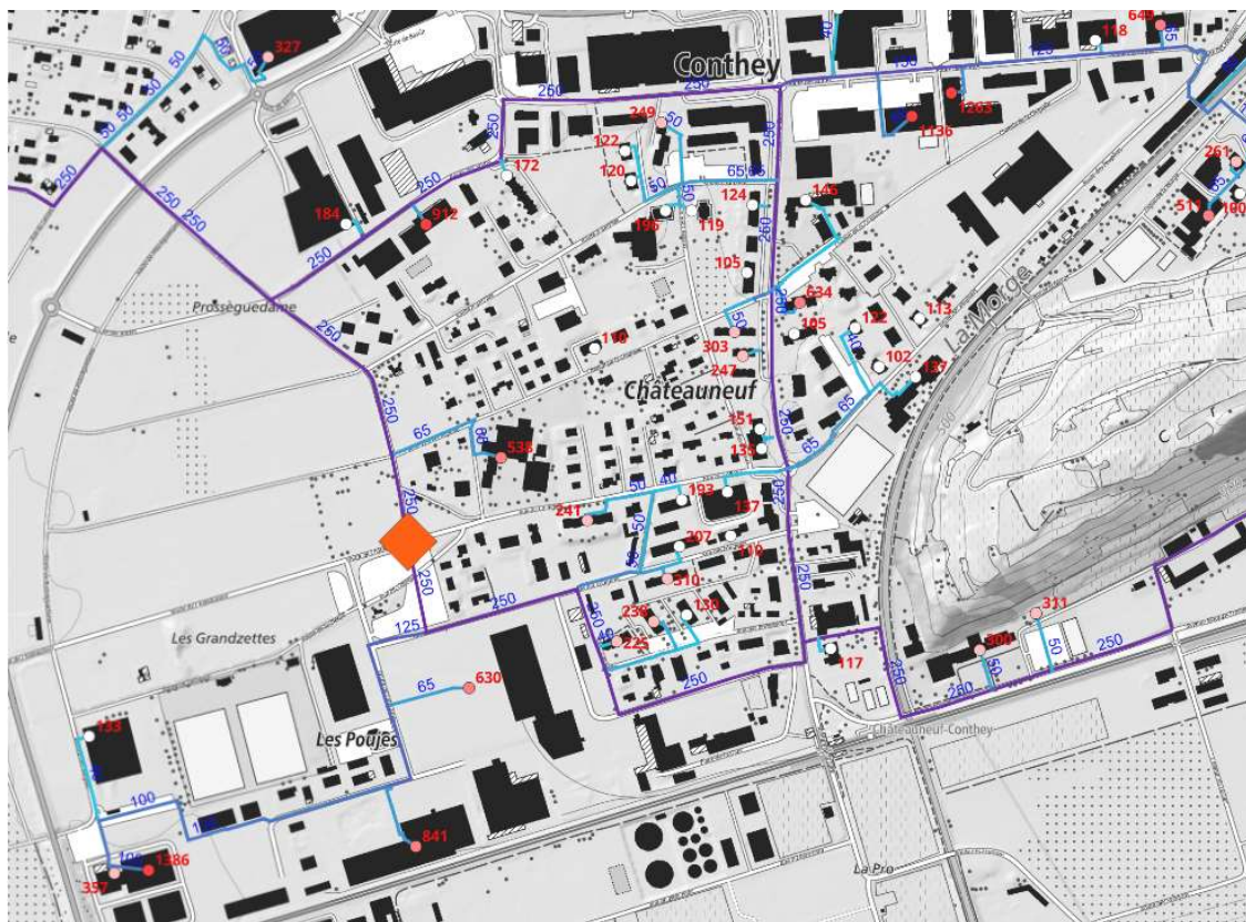
Figure 2: Dimensionnement du réseau
